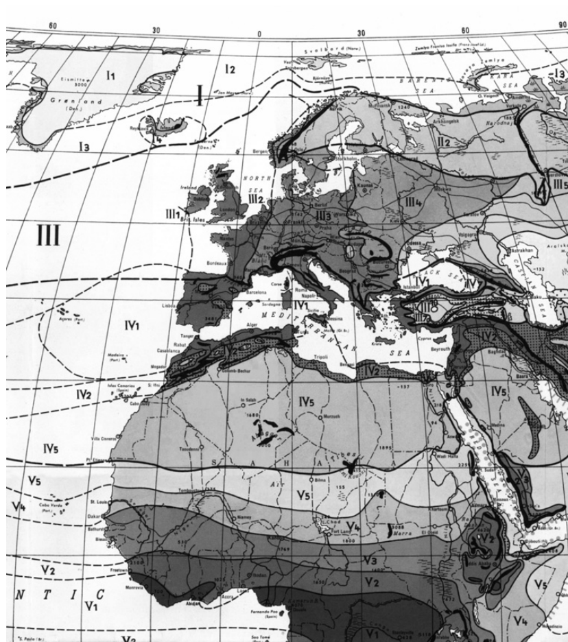
Figure 1.2 Detail of Troll and Paffen's "Seasonal Climates of the Earth." C. Troll, "Karte der Jahreszeitenklima der Erde, mit einer farbigen Karte von C. Troll und K. H. Paffen," Erdkunde 18 (1964): 5–28. By permission of Erdkunde .
