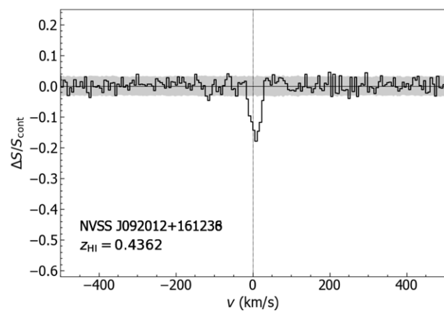
15. NVSS J092012+161238
