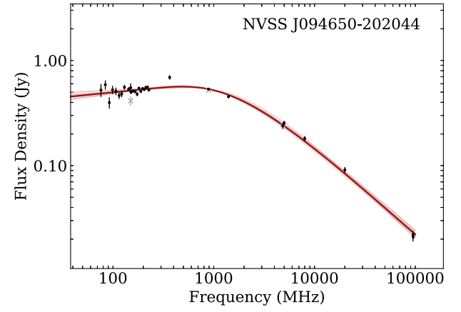
16. NVSS J094650-202044
