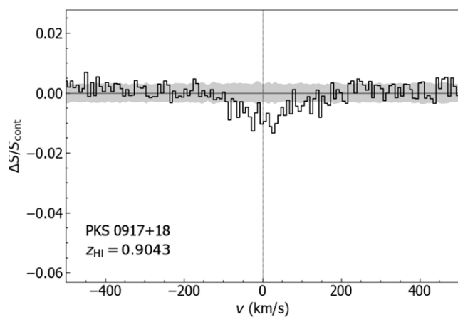
13. NVSS J091256+030021
