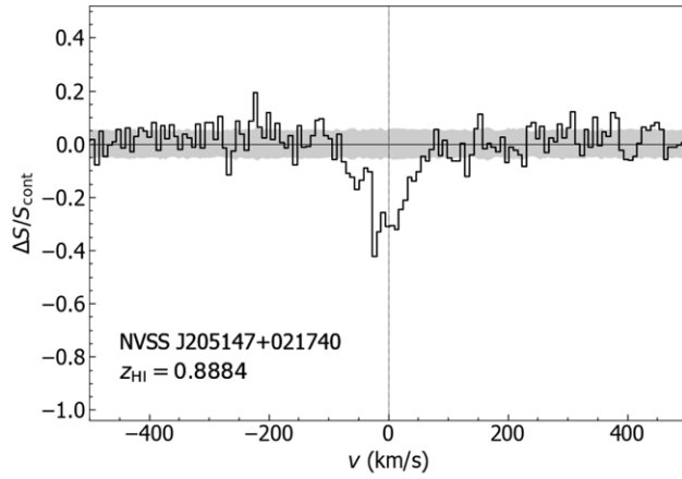
22. NVSS 205147+021740
