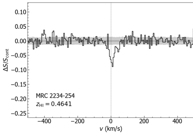
27. MRC 2234-254
