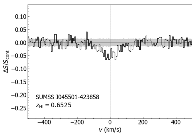
8. SUMSS J045501-423858
