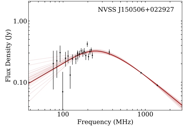
19. NVSS J150506+022927
