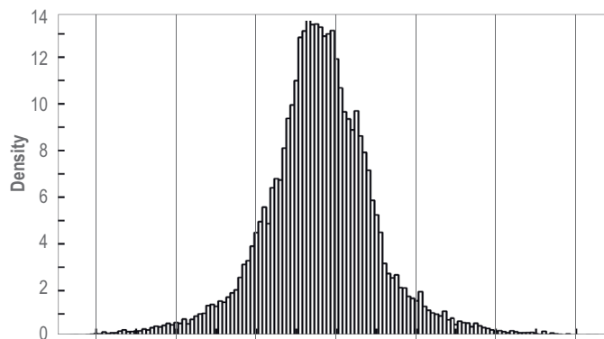
(d) SSP5-8.5
