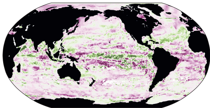
(a) SSP1-2.6
